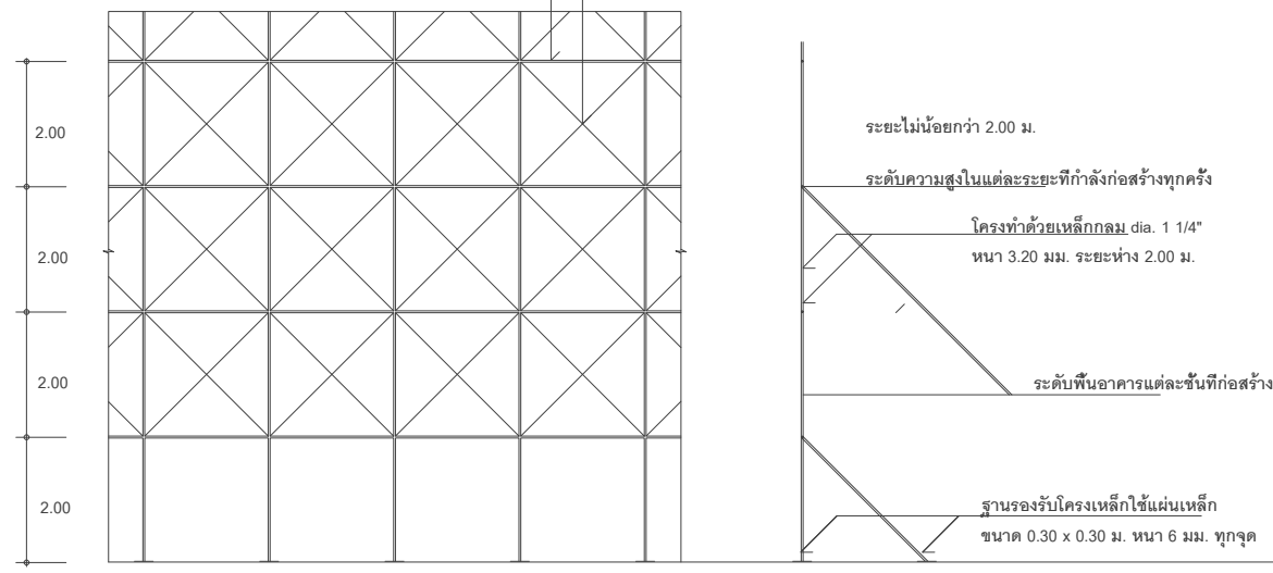
แบบขยายรูปด้านตั้งด้านหน้า
